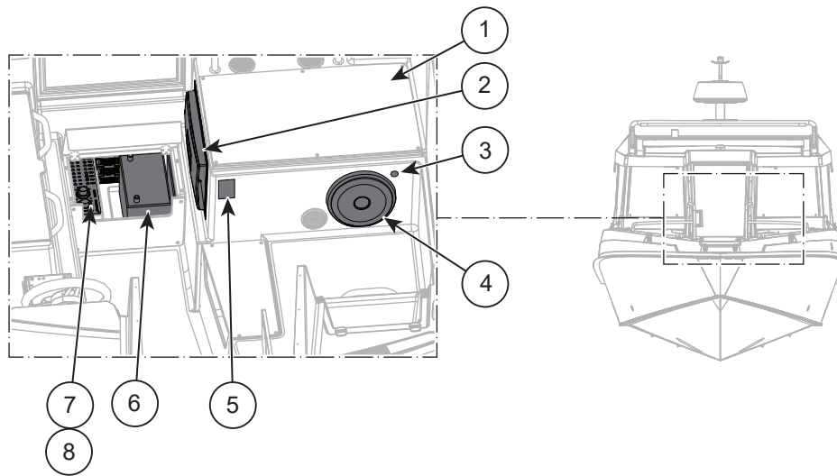
Kuva 8.2 Kajuutan näkymä
