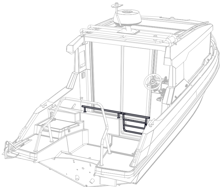
Kuva 4.2 Buster Magnum Cabin kulkuportti
