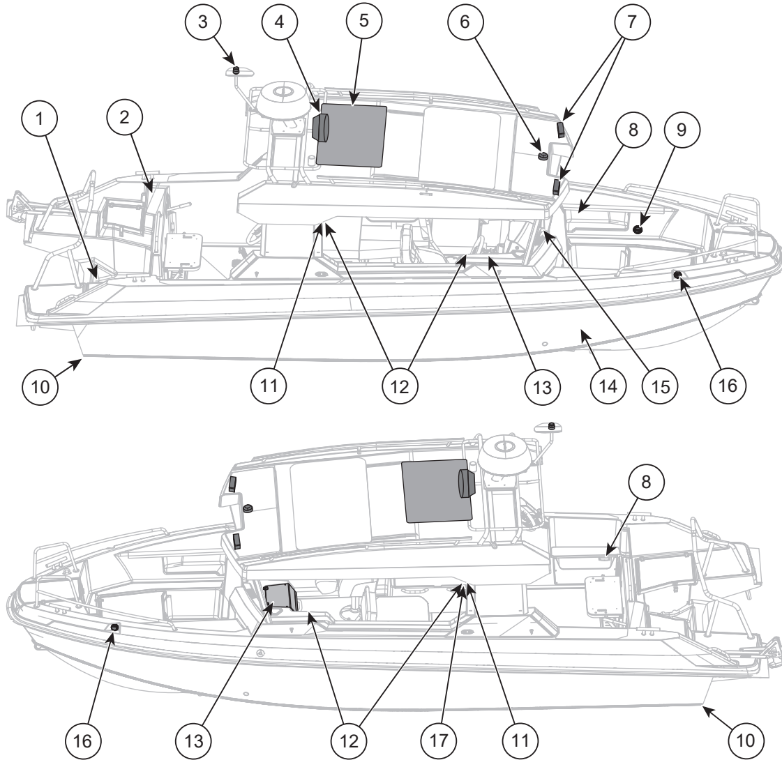
Kuva 8.3 Sivunäkymä
