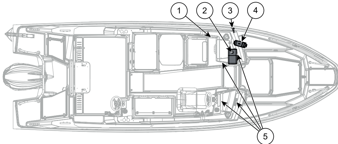
Kuva 6.2 Lämmitinjärjestelmän komponentit
