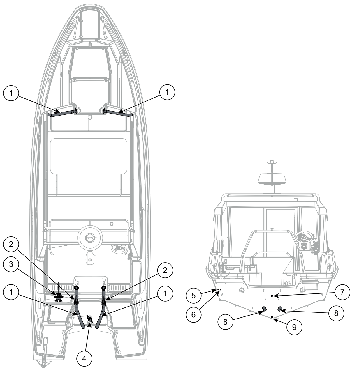
Kuva 9.1 Buster Magnum Cabin tyhjennysvarusteet
