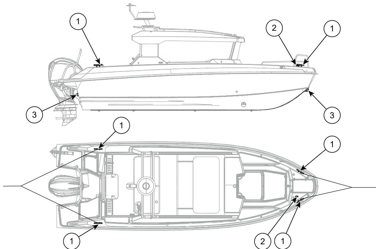
Kuva 5.7 Buster Magnum Cabin kiinnitys- ja hinauspisteet
