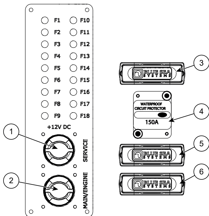
Kuva 8.1 Buster Magnum Cabin päävirtakytkimet ja sulakepaneeli
