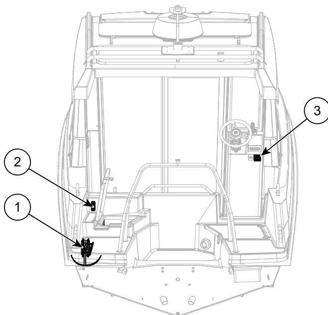
Kuva 10.1 Buster Magnum Cabin ankkurivinssi
