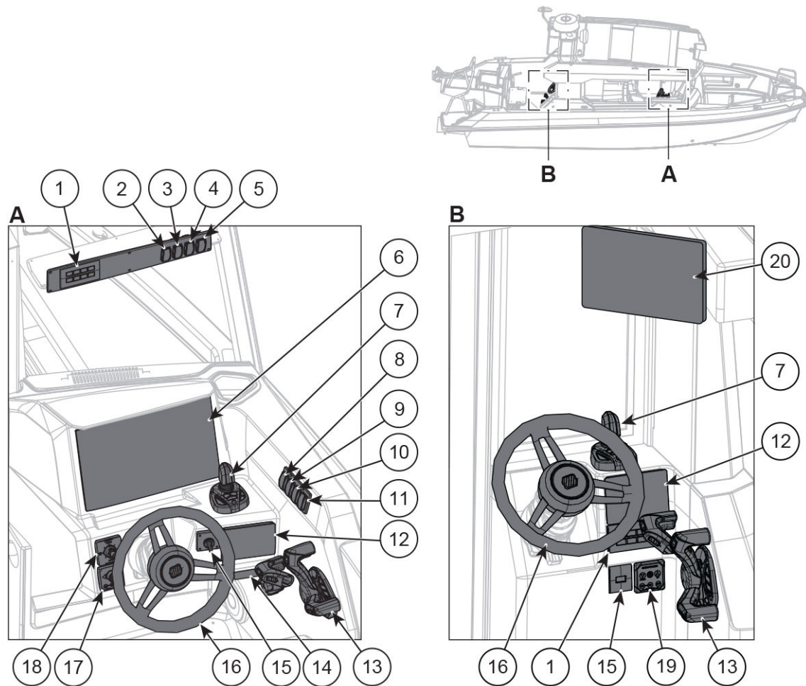
Kuva 5.1 Kajuutan ohjauspisteen hallintalaitteet (A) ja valinnaisen ulko-ohjauspisteen (B) hallintalaitteet
