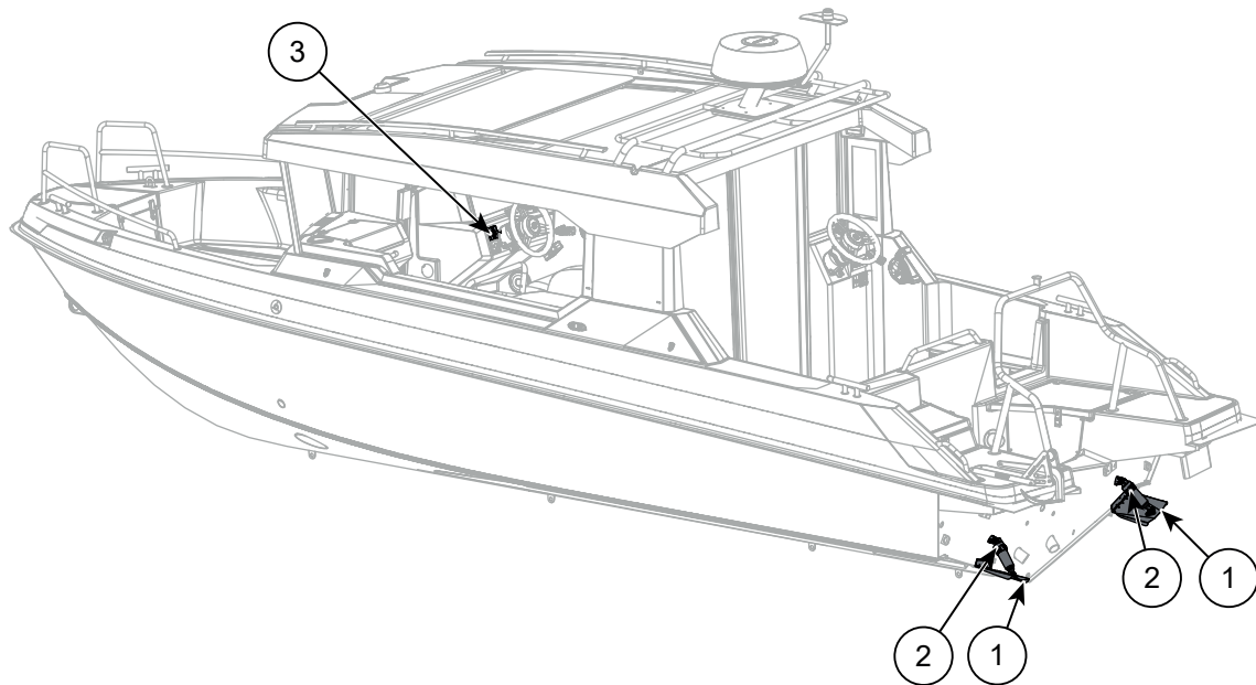
Kuva 5.6 Trimmijärjestelmän komponenttien sijainti
