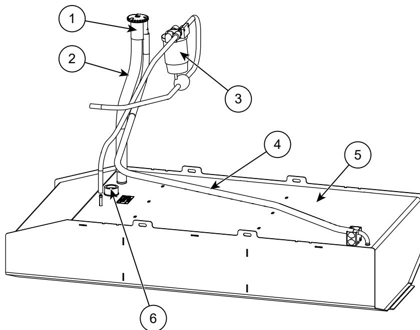
Kuva 6.1 Polttoainejärjestelmä
